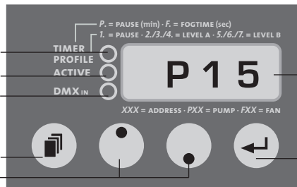
Fig. 1: Réglage du débit de la pompe
