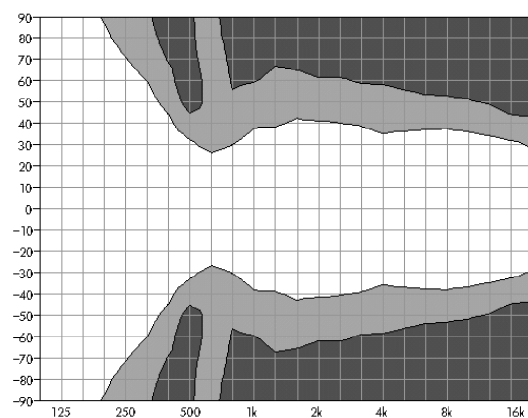
Fig. 7: Diagramme isobare Q7 horizontal, configuration horizontale avec pavillon tourné
