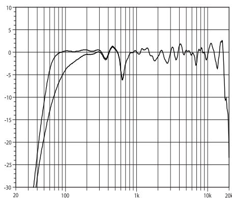
Fig. 9: Réponse en fréquence de la Q7, modes standard et CUT
