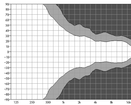
Fig. 8: Diagramme isobare Q7 vertical, configuration horizontale avec pavillon tourné
