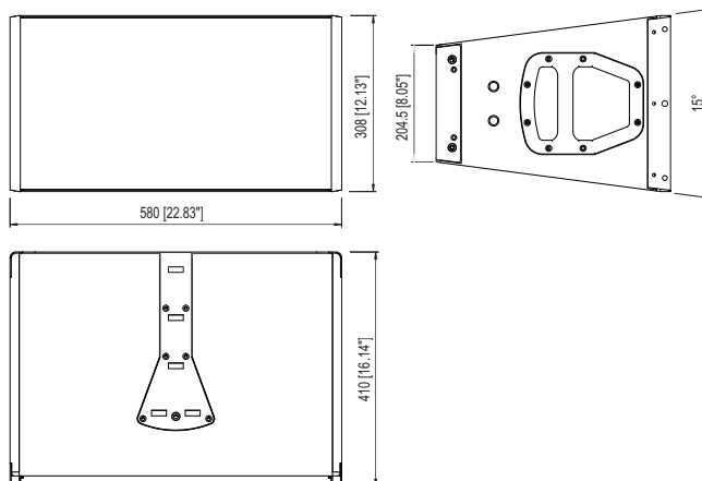
Fig. 10: Q7 dimensions du coffre en mm [inch]
