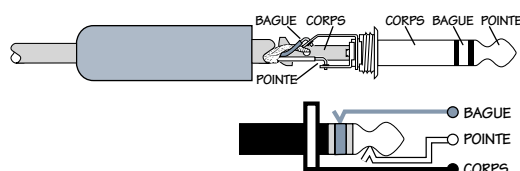
Figure B : Jack 6,35 mm stéréo
